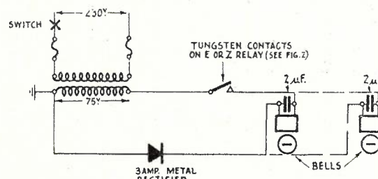
Fig. 4.—Bell Circuits.
